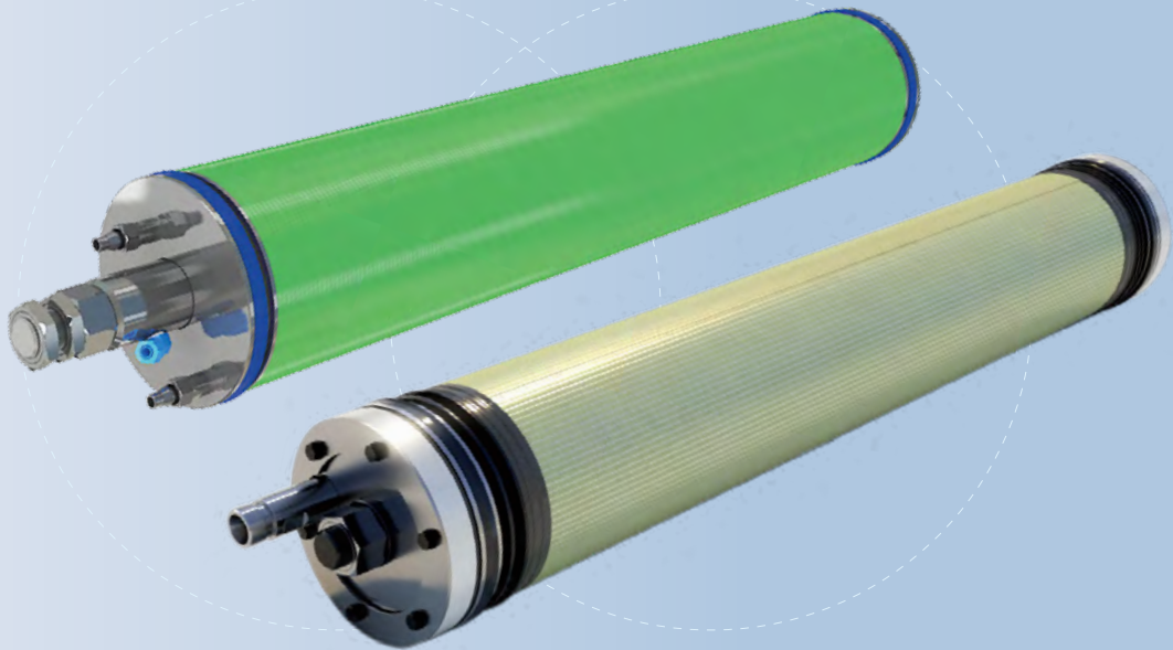
DT/ST 膜组件
